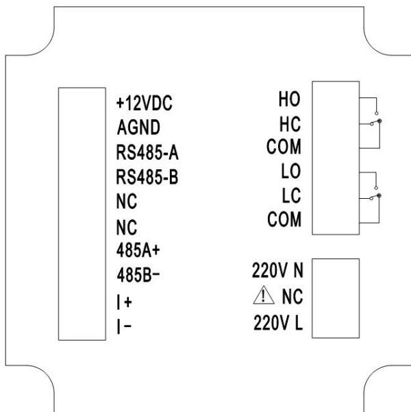
图 5 接线图
