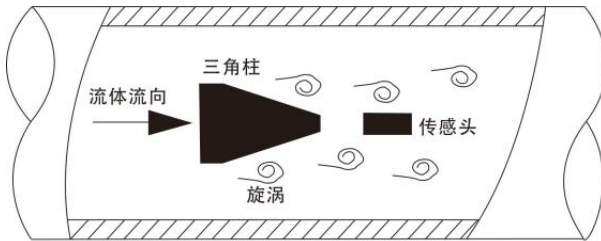
图 1 涡街流量计
