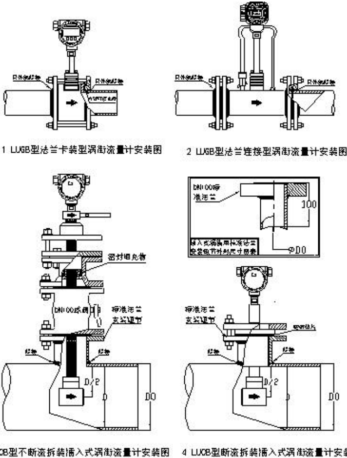
图4 LUGB型、LUCB型涡街流量计安装及焊接示意图
