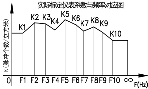
图 13 实际标定仪表系数与频率对应图
