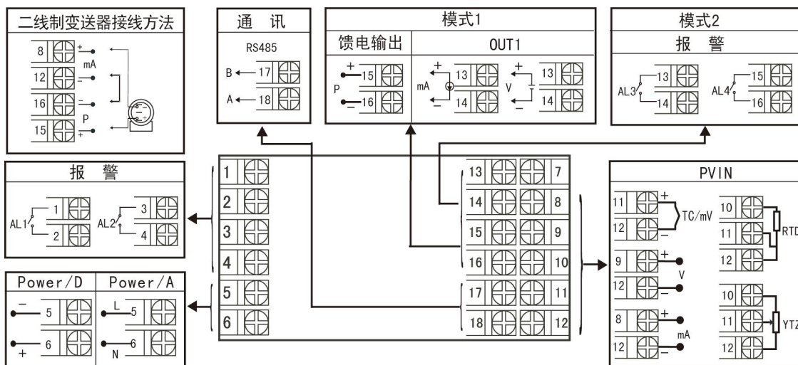
图 8 规格尺寸为 H 型接线图
