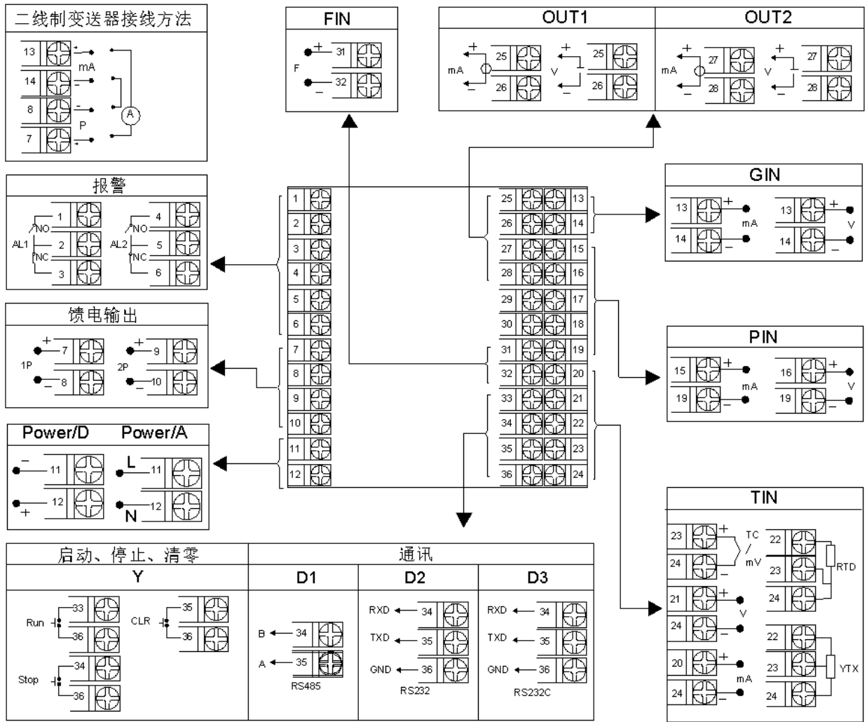
图 13 规格尺寸为 A、B、C、D 型接线图
