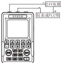
图 3 二线制变送器模拟器
