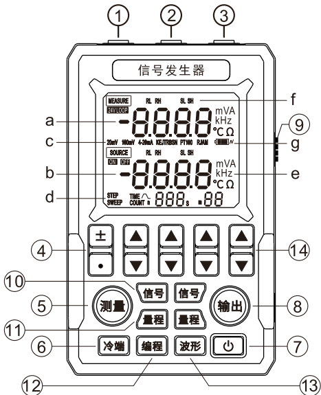
图 1 信号发生器正视图
